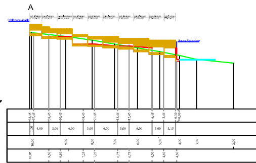
Profilo longitudinale A-B \nabla +0,00 Distanze Progressive Distanze Parziali Quote Terreno Quote Progetto
