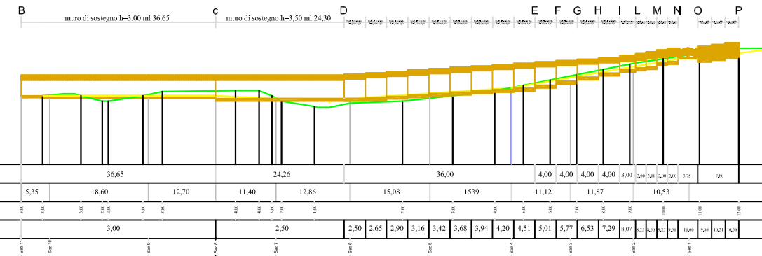
Profilo longitudinale \nabla -10,00 Distanze Parziali Distanze Parziali Sezioni Quote Terreno Quote Progetto muro N. sezioni trasversali
